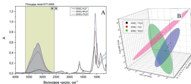
Рисунок 1. А: Расчёт площади пика под кривой образца \text{ZnSO}_4 \cdot 7\text{H}_2\text{O} . В: 3D-МГК для области ИК-спектров, соответствующей колебанию гидроксильной группы (3635 - 2568 \text{cm}^{-1} ).
