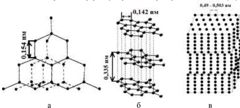
Рис. 1. Пример, как структура кристаллической решетки: а) алмаза; б) графита; в) карбина, меняет их свойства в пространстве.
