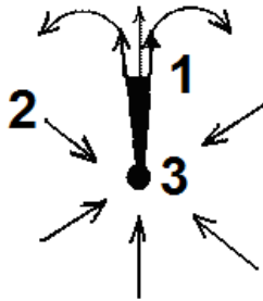
Рис. 5. Классическая схема формирования кумулятивной струи и джета (1) при коллапсе энергомассовоимпульсных потоков (2) в аттрактор (3). Выброс кумулятивной струи и формирование джета происходит в ослабленной, например, внешним воздействием, области аттрактора.
