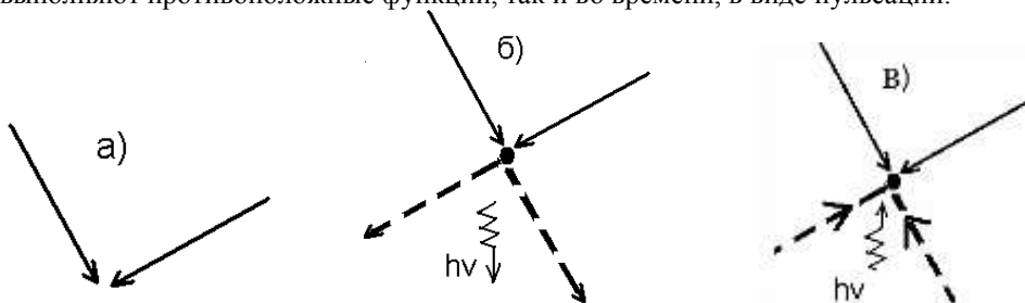
Рис. 2. Схема: а) кумуляции (схождения) энергомассовоимпульсных потоков; б) кумуляции и диссипации ЭМИП, в том числе и через излучение электромагнитных вол с энергией h\nu ; в) кумуляции массы и энергии. Точка – узел или перетяжка ЭМИП в сформировавшейся КД-структуре.
