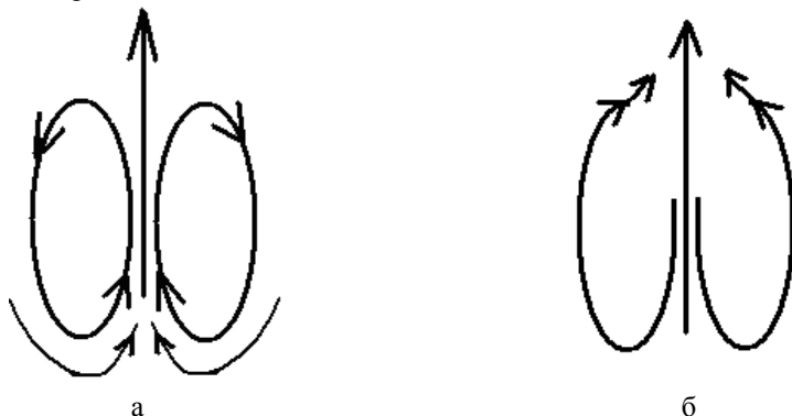
Рис. 4. Элементарная схема самоорганизующейся: а) энергосберегающей кумулятивно-диссипативной смерчеобразной структуры – «свечи» с областью кумуляции ЭМИП (внизу) и кумулятивной струей (вверху), пробивающей любую броню; б) самоуничтожающейся структуры, когда все потоки работают только на вынос ЭМИП из структуры, например, выносят капитал из государства с «зоо»-кратией в другую социальную разумно организованную структуру (рис. 4 а).
